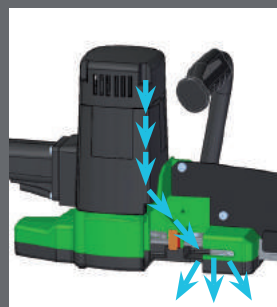
Λειτουργία ανεμιστήρα
