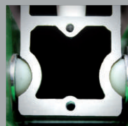
BST 182 V/S: κίνηση φορείου σε 4 ειδικές σφαίρες
